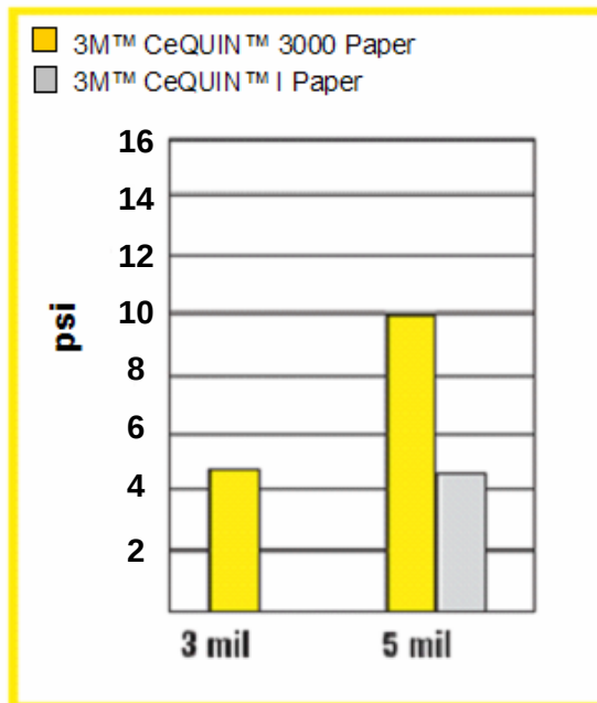
MULLEN BURST
