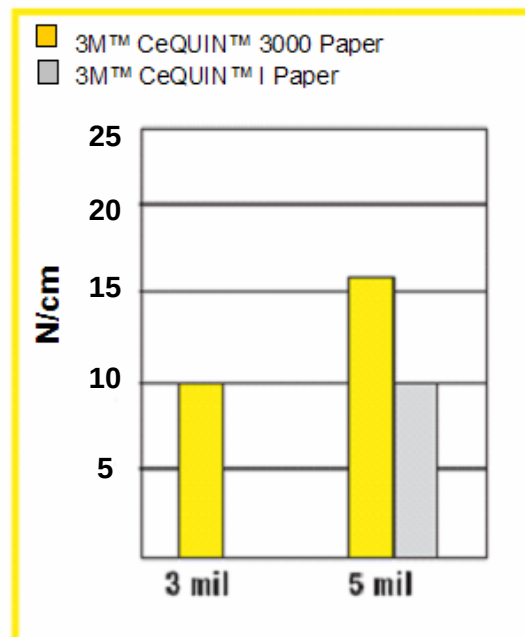
TENSILE STRENGTH
